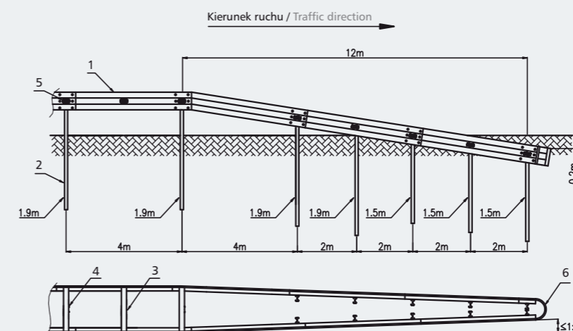
Przykładowe zakończenie systemu H1 W6 (SP-07/4) Example of terminal for system H1 W6 (SP-07/4)
