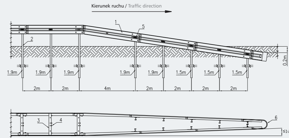
Przykładowe zakończenie dla systemu H1 W5 (SP-07/2) Terminal for system H1 W5 (SP-07/2)
