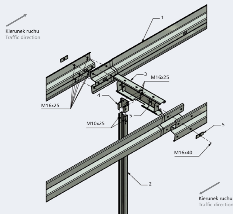
Schemat montażowy bariery SP-07/2 Assembly of barrier SP-07/2
