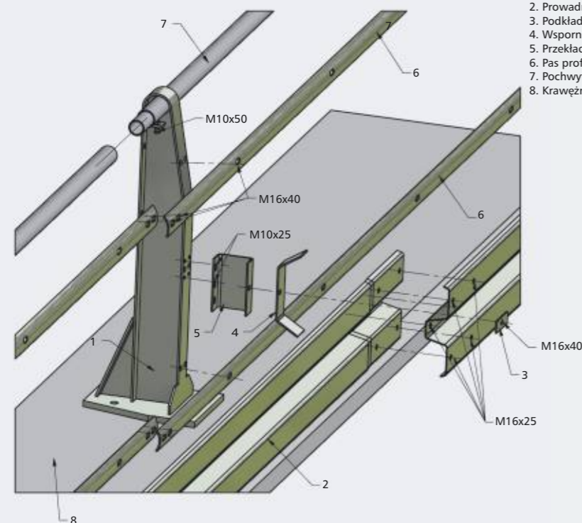
Schemat montażowy bariery BSP-160K/1.33 Assembly of barrier BSP-160K/1.33
