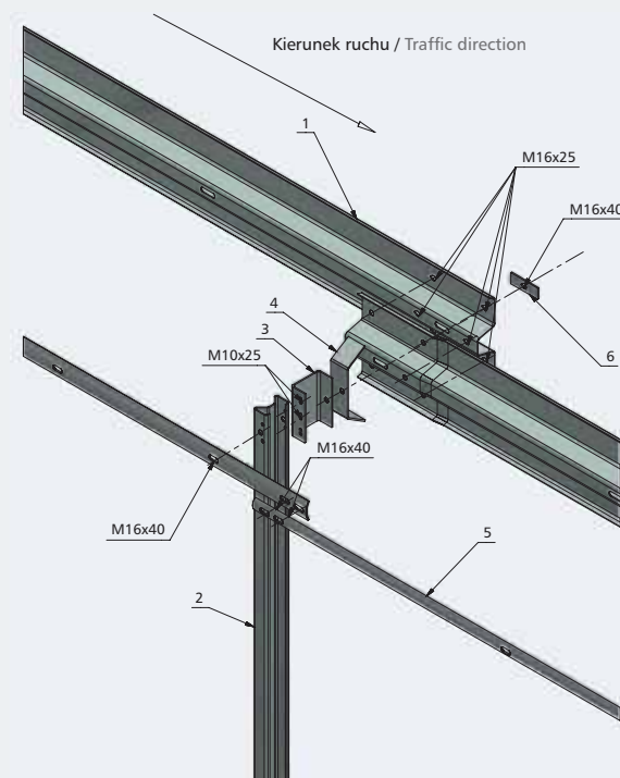
Schemat montażowy systemu N2 W5 (SP-09/4) Assembly of system N2 W5 (SP-09/4)
