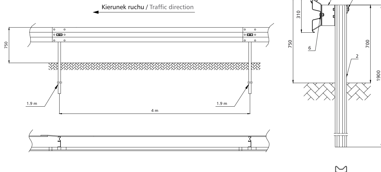
Lista elementów: / List of elements: 1. Prowadnica B / Guardrail Type B 2. Słupek Sigma / Sigma Post 3. Przekładka C120 / Spacer C120 4. Pas profilowy / Shaped Belt 5. Wspornik B / Bracket Type B 6. Podkładka M16 / Washer M16
