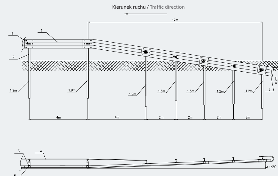
Zakończenie systemu SP-09/4 Terminal for system SP-09/4
