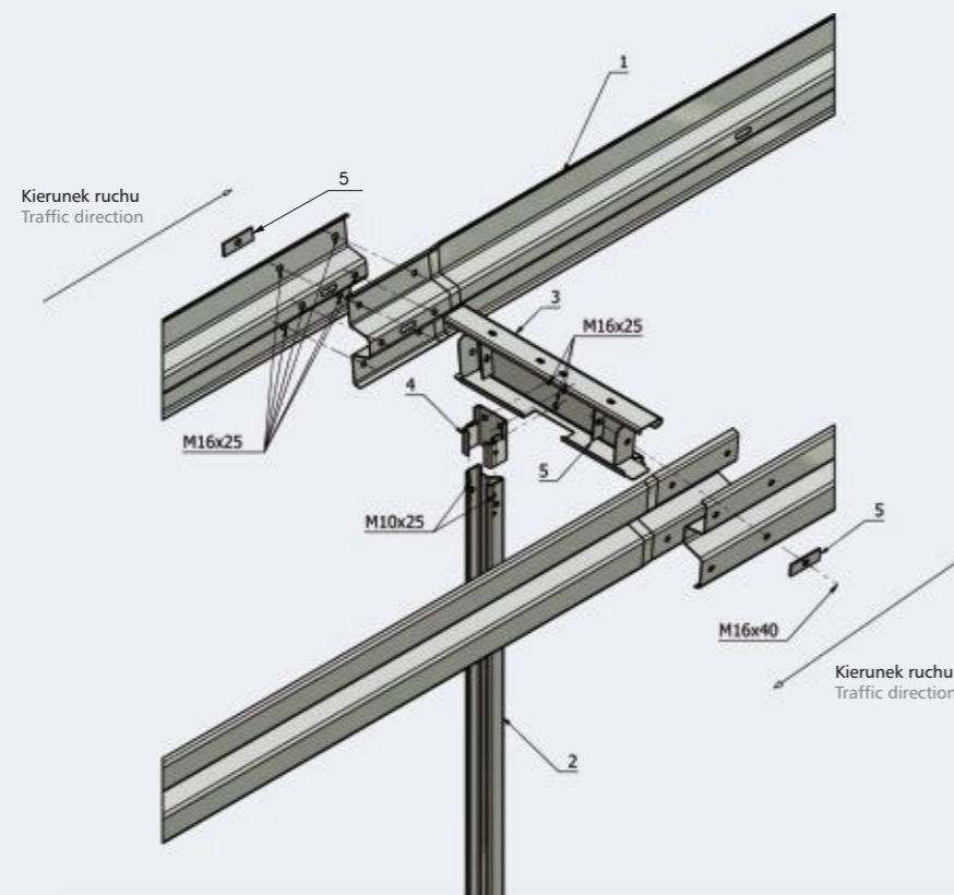
Schemat montażowy bariery SP-07/1.33 Assembly of barrier SP-07/1.33
