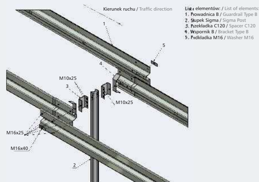
Schemat montażowy systemu N2 W6 (SP-10/4) Assembly of system N2 W6 (SP-10/4)
