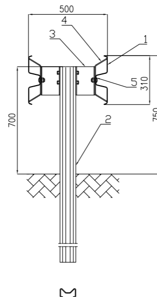
Lista elementów: / List of elements: 1. Prowadnica B / Guardrail Type B 2. Słupek Sigma / Sigma Post 3. Przekładka C120 / Spacer C120 4. Wspornik B / Bracket Type B 5. Podkładka M16 / Washer M16
