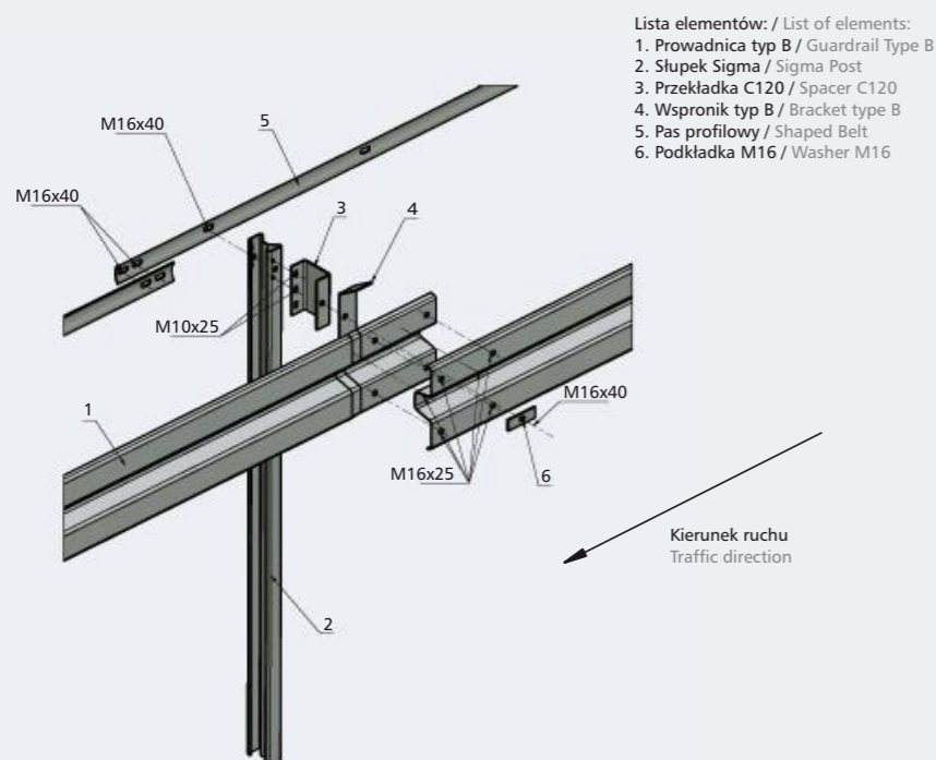
Schemat montażowy bariery SP-09/2 Assembly of barrier SP-09/2
