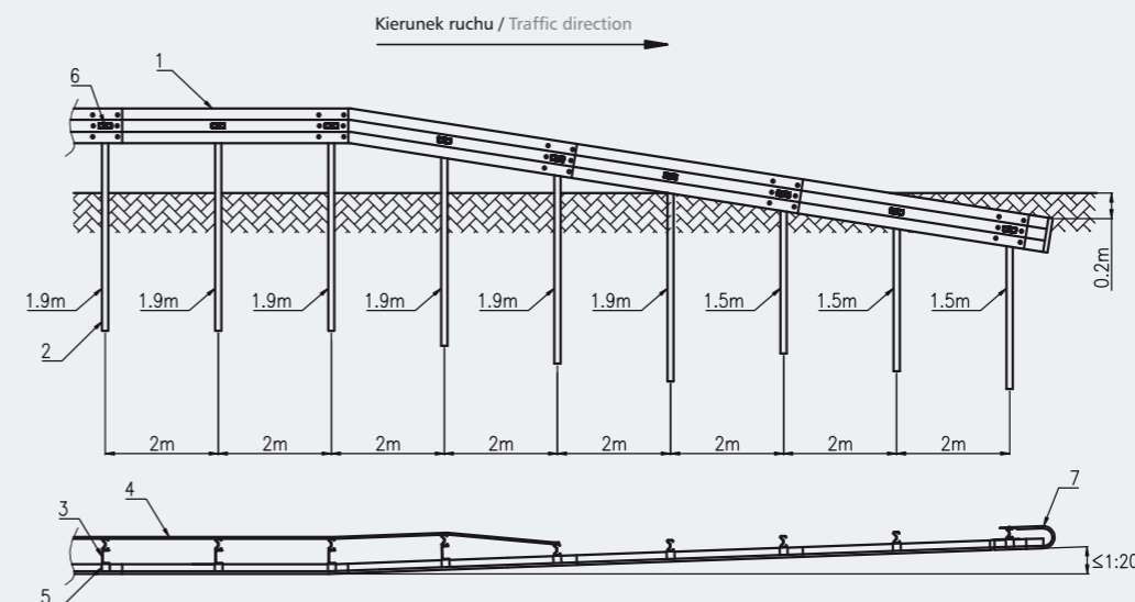
Przykładowe zakończenie systemu H1 W6 (SP-09/2) Example of terminal for system H1 W6 (SP-09/2)
