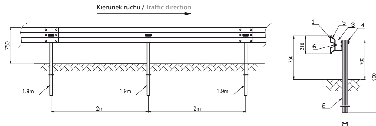
Lista elementów: / List of elements: 1. Prowadnica B / Guardrail Type B 2. Słupek Sigma / Sigma Post 3. Przekładka C120 / Spacer C120 4. Pas profilowy / Shaped Belt 5. Wspronik typ B / Bracket type B 6. Podkładka M16 / Washer M16
